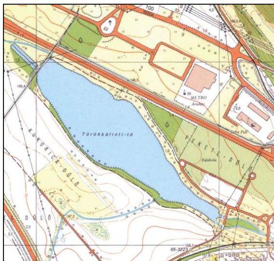
ábra A Sasad I. tározó (Törökbálinti-tó) áttekintő helyszínrajza
