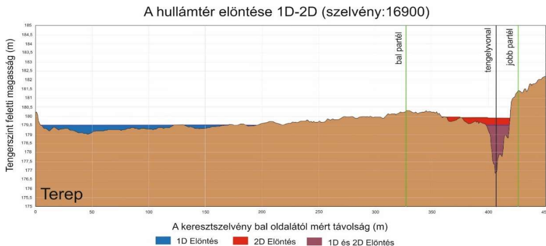
18. ábra Eltérés a teljes 1D és teljes 2D geometriai kialakítás előntési eredményei közt az Eger-patak 16+900 kereszt-szelvényénél. A 2D kialakítás esetében a víz a mederben marad, míg az 1D modell eredményei hibás előntést mutatnak a vízfolyás bal oldalán fekvő síkvidéki területen.
