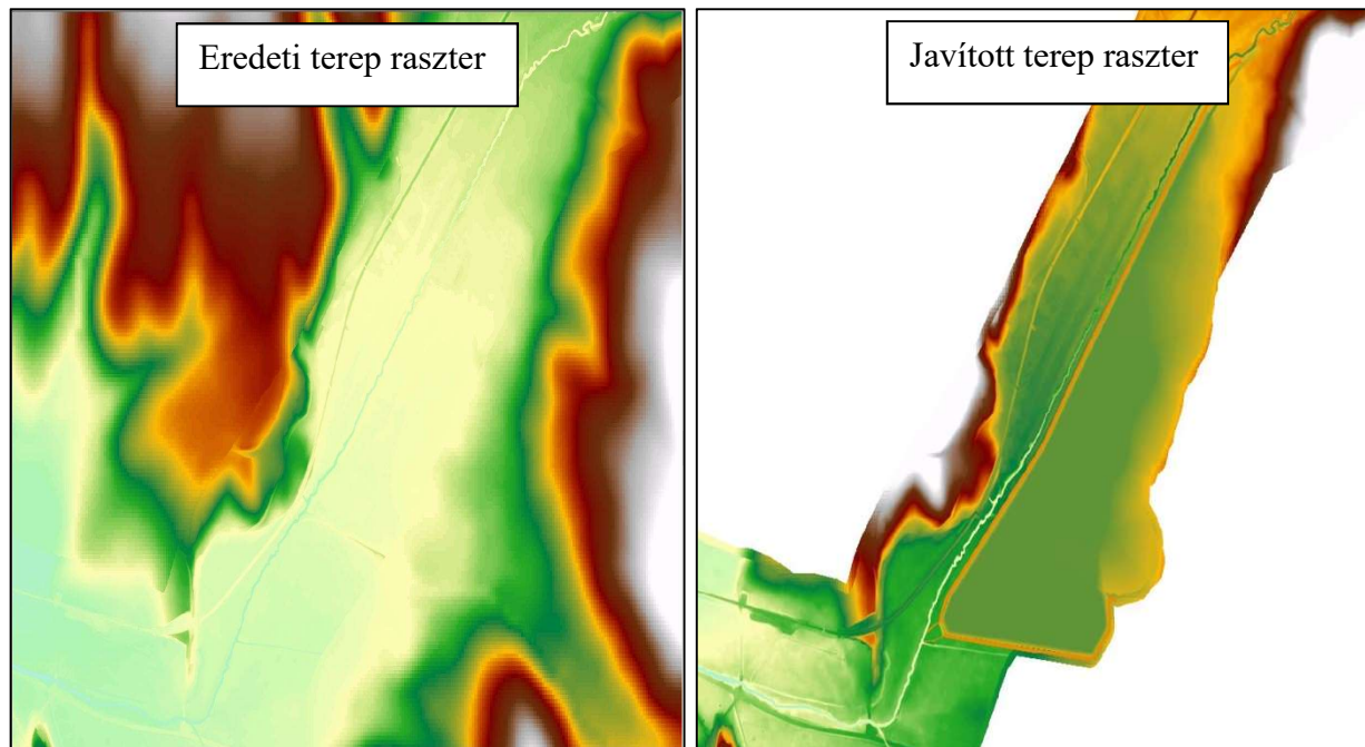
19. ábra. A Magyarszéki tározó beégetése a Baranya-csatorna modellezéshez használt terep raszterbe. A Baranya-csatornán a többi vízfolyással ellentétben a kvázi permanens állapot helyett árhullámot futtattunk, hogy vizsgálni tudjuk a tározó hatását az elöntésre.
