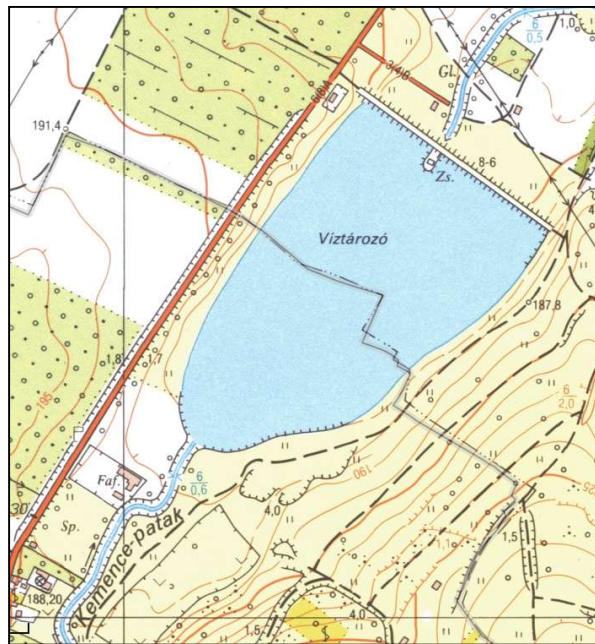
ábra A Kemence pataki tározó áttekintő helyszínrajza
