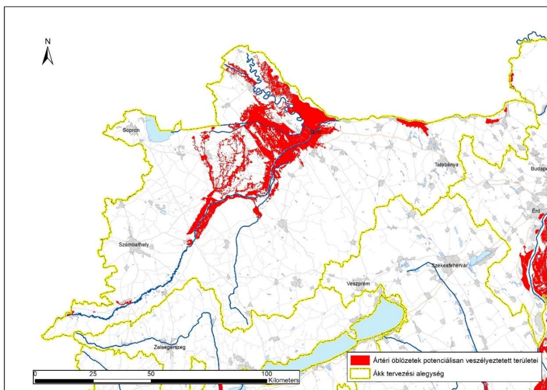
15. ábra Az ártéri öblözetek előzetes kockázatbecslés során megállapított potenciálisan veszélyeztetett területei
