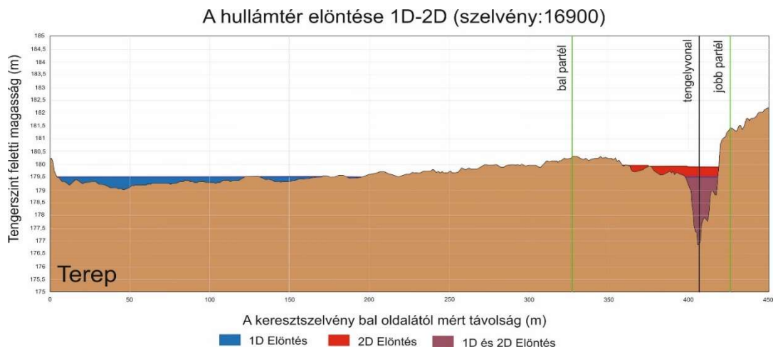
18. ábra Eltérés a teljes 1D és teljes 2D geometriai kialakítás elöntési eredményei közt az Eger-patak 16+900 keresztmetszvényénél. A 2D kialakítás esetében a víz a mederben marad, míg az 1D modell eredményei hibás elöntést mutatnak a vízfolyás bal oldalán fekvő síkvidéki területen.
