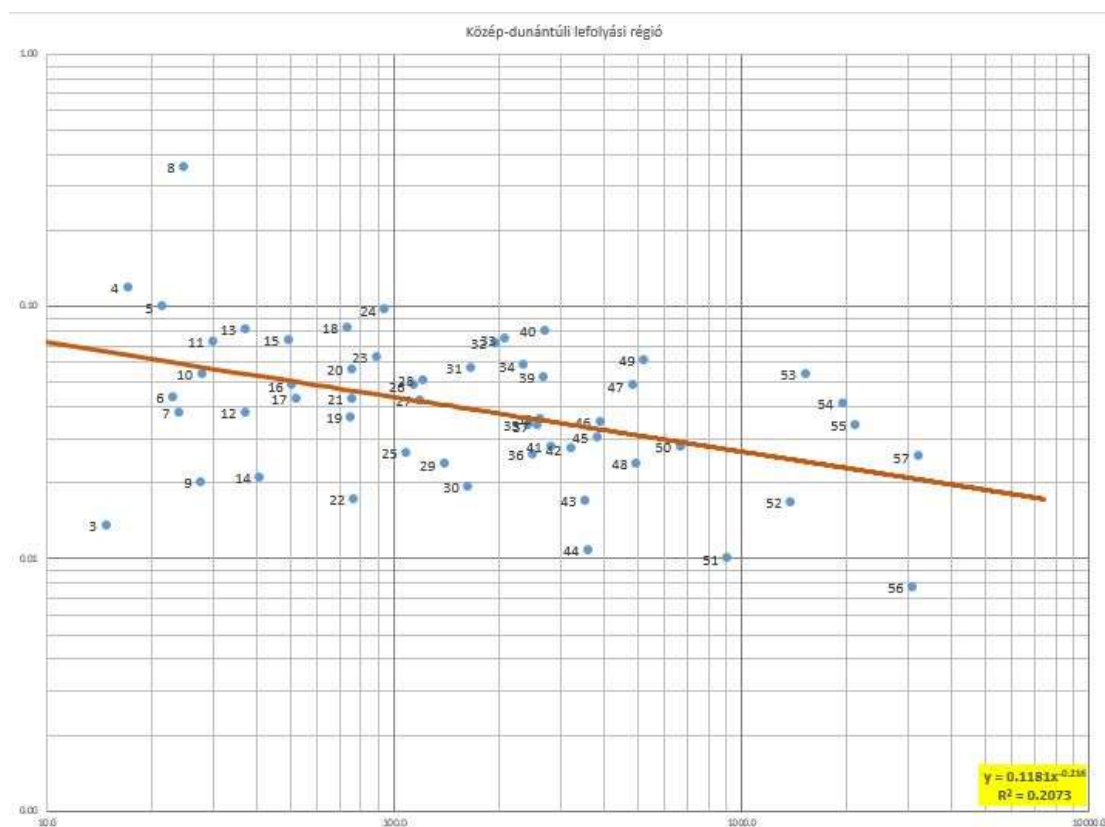
21. ábra A Közép-dunántúli lefolyási régió számítási függvénye. Az 57 vízmércéhez tartozó 5%-os fajlagos árvízhozam érték. A tanulmányt megalapozó vízmérce idősorok jóval megbízhatóbb statisztikai alapadatként szolgálnak a korábban használt adatoknál. A tanulmányhoz készült adatbázis folyamatos frissítésével a későbbiekben egyre pontosabb input vízhozam adatokkal láthatjuk el a kész kisvízfolyás modelleket.
