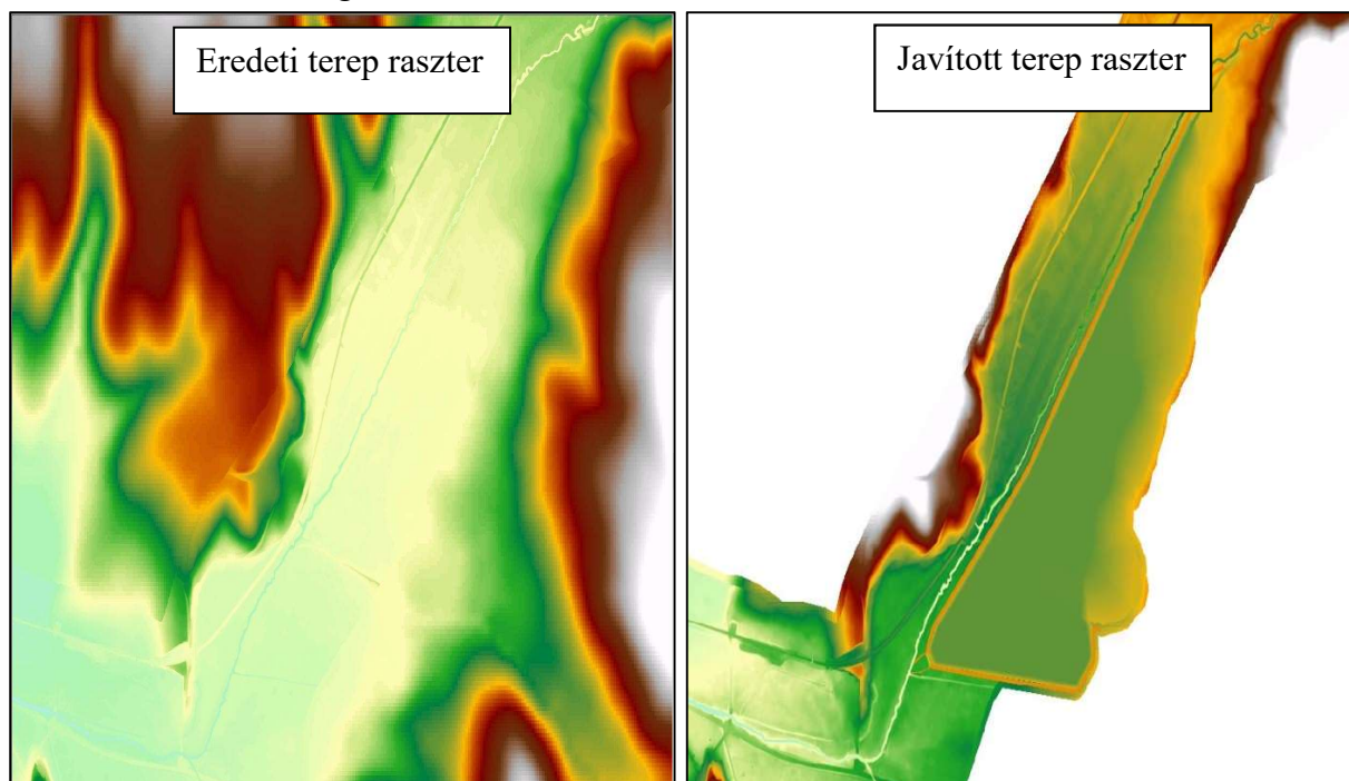
19. ábra. A Magyarszéki tározó beégetése a Baranya-csatorna modellezéshez használt terep raszterbe. A Baranya-csatornán a többi vízfolyással ellentétben a kvázi permanens állapot helyett árhullámot futtattunk, hogy vizsgálni tudjuk a tározó hatását az elöntésre.
