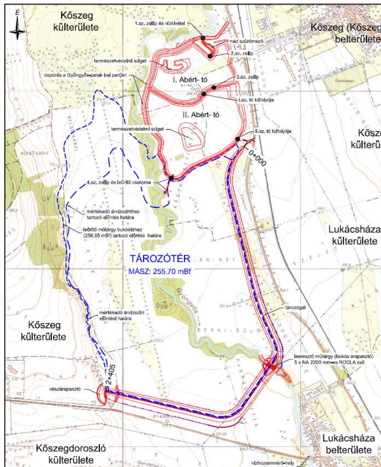
3. ábra Lukácsházi árvízcsúcs-csökkentő tározó átnézetes helyszínrajza
