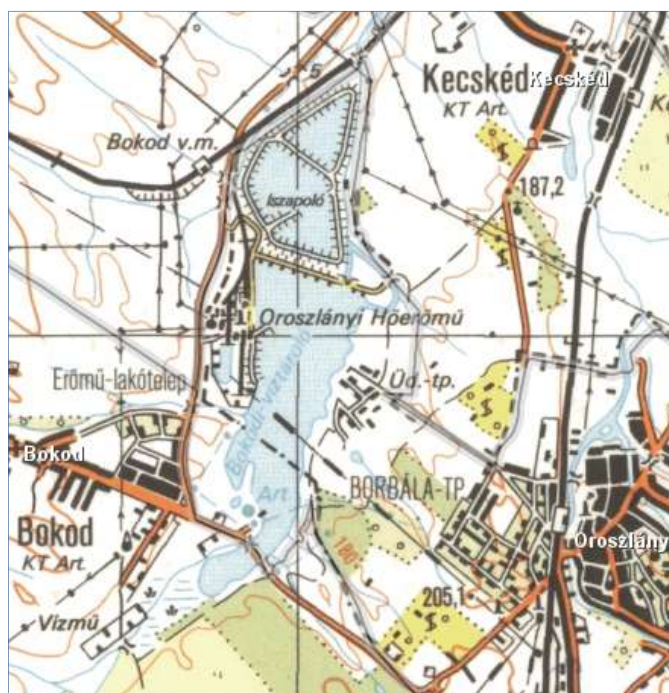
6. ábra Bokodi hűtőtó áttekintő helyszínrajza
