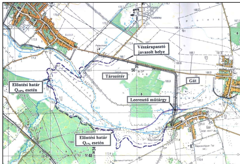
4. ábra Góri tározó átnézetes helyszínrajza
