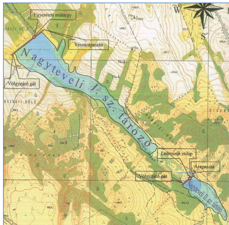
5. ábra Nagyteveli I. és II. tározó helyszínrajza
