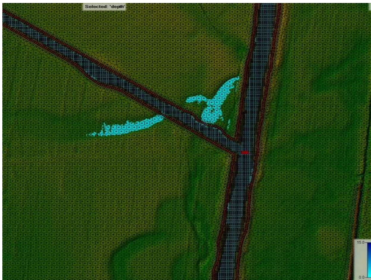
20. ábra Végeges HEC-RAS 2D modell geometriai kialakítás a Babócsai-Rinya vízfolyás esetében. A főmeder, és a töltésezett betorkolló vízfolyások medrek esetében területi rácsháló sűrítést alkalmaztunk. A magaspontok geometriába építésével sikeresen integráltuk a vízterelők elöntésre gyakorolt hatását a modellekbe. A meder esetében négyszög, az ártér esetében hatszög alakú rácshálót hoztunk létre.
