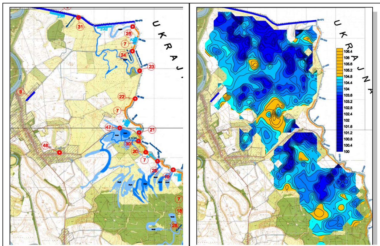
5. ábra A Lónyai fióktározó átnézeti helyszínrajza árvízi és természetvédelmi vízpótlás esetén
