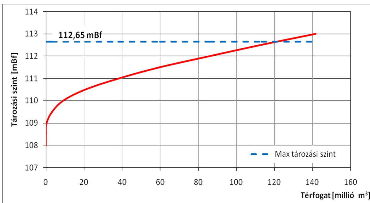
7. ábra A Szamos-Krasznaközi árapasztó tározó térfogati görbéje
