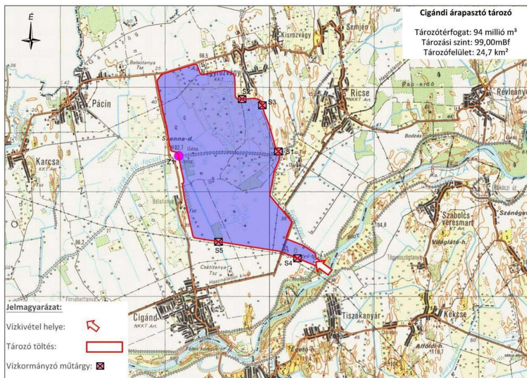
8. ábra A Cigándi árapasztó tározó átnézetes helyszínrajza
