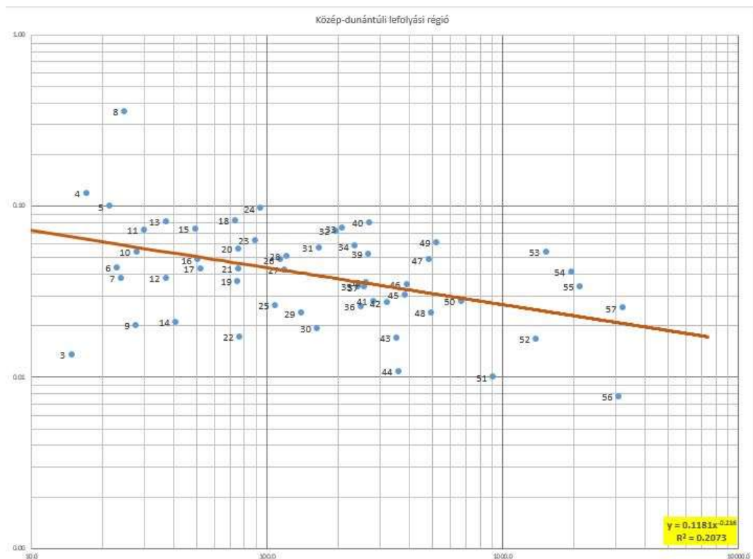
23. ábra A Közép-dunántúli lefolyási régió számítási függvénye. Az 57 vízmércéhez tartozó 5%-os fajlagos árvízhozam érték. A tanulmányt megalapozó vízmérce idősorok jóval megbízhatóbb statisztikai alapadatként szolgálnak a korábban használt adatoknál. A tanulmányhoz készült adatbázis folyamatos frissítésével a későbbiekben egyre pontosabb input vízhozam adatokkal láthatjuk el a kész kisvízfolyás modelleket.
