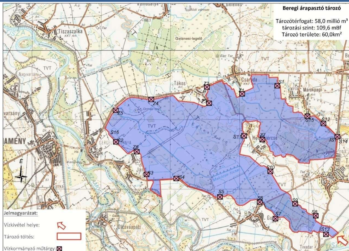
3. ábra A Beregi tározó átnézetes helyszínrajza
