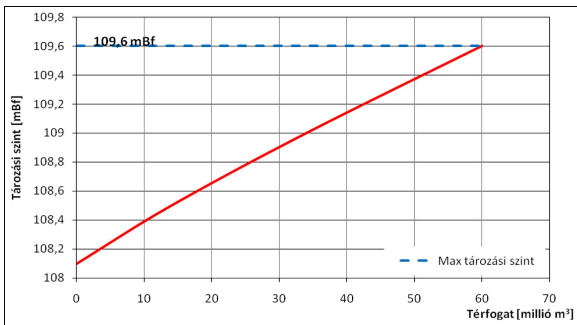
4. ábra A Beregi árapasztó tározó térfogati görbéje
