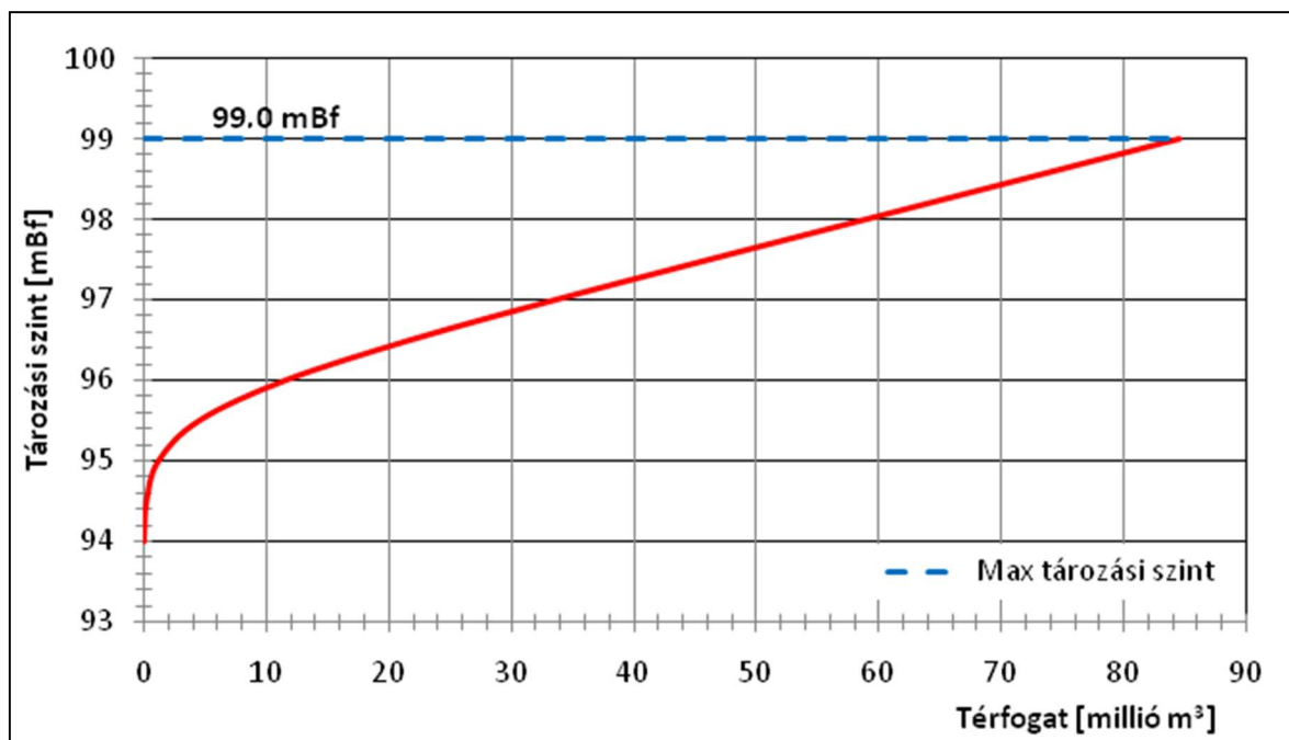
9. ábra A Cigándi árapasztó tározó térfogati görbéje
