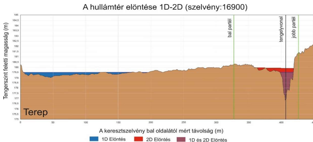
20. ábra Eltérés a teljes 1D és teljes 2D geometriai kialakítás elöntési eredményei közt az Eger-patak 16+900 keresztmetszvényénél. A 2D kialakítás esetében a víz a mederben marad, míg az 1D modell eredményei hibás elöntést mutatnak a vízfolyás bal oldalán fekvő síkvidéki területen.
