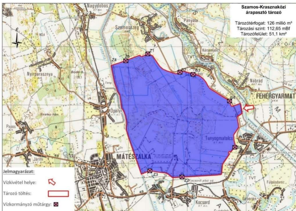
6. ábra A Szamos-Krasznaközi tározó átnézetes helyszínrajza
