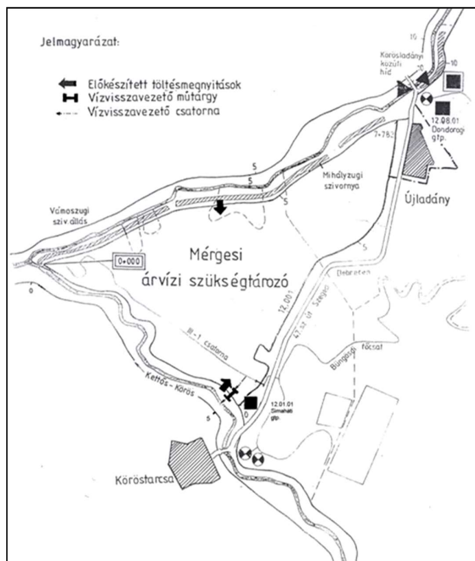
7. ábra A Mérgesi tározó átnézeti helyszínrajza (Galbáts et al., 2004)
