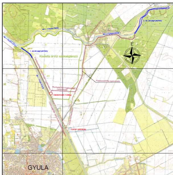
6. ábra A Kisdelta árvízszükségeltározó áttekintő helyszínrajza (Konstruktőr Kft.)
