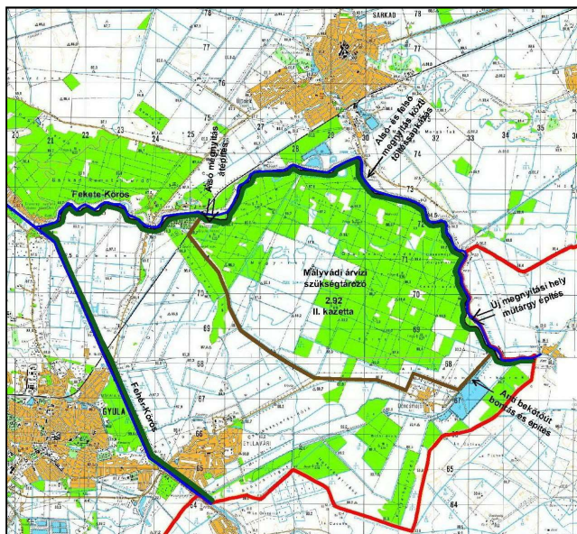
5. ábra A Mályvádi árvízszükségeltározó áttekintő helyszínrajza (KÖVIZIG)
