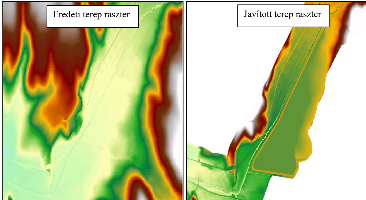
20. ábra. A Magyarorszáki tározó beégetése a Baranya-csatorna modellezéshez használt terep raszterbe. A Baranya-csatornán a többi vízfolyással ellentétben a kvázi permanens állapot helyett árhullámot futtattunk, hogy vizsgálni tudjuk a tározó hatását az előntésre.
