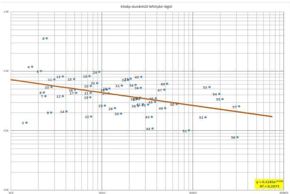
22. ábra A Közép-dunántúli lefolyási régió számítási függvénye. Az 57 vízmércéhez tartozó 5%-os fajlagos árvízhozam érték. A tanulmányt megalapozó vízmérce idősorok jóval megbízhatóbb statisztikai alapadatként szolgálnak a korábban használt adatoknál. A tanulmányhoz készült adatbázis folyamatos frissítésével a későbbiekben egyre pontosabb input vízhozam adatokkal láthatjuk el a kész kisvízfolyás modelleket.
