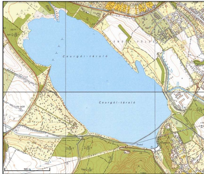
3. ábra A Fehérvárcsurgói tározó áttekintő helyszínrajza
