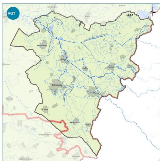
Délkelet-Alföld porózus termál felszín alatti víztest
