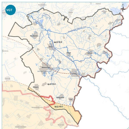
Körös-Maros köznevi sekély porózus felszín alatti víztest
