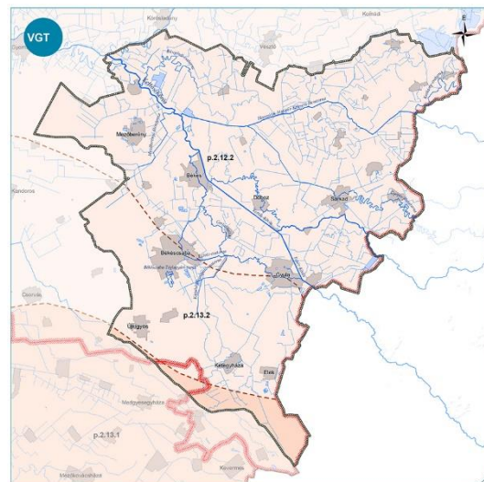
Körös-Maros köznevi porózus felszín alatti víztest
