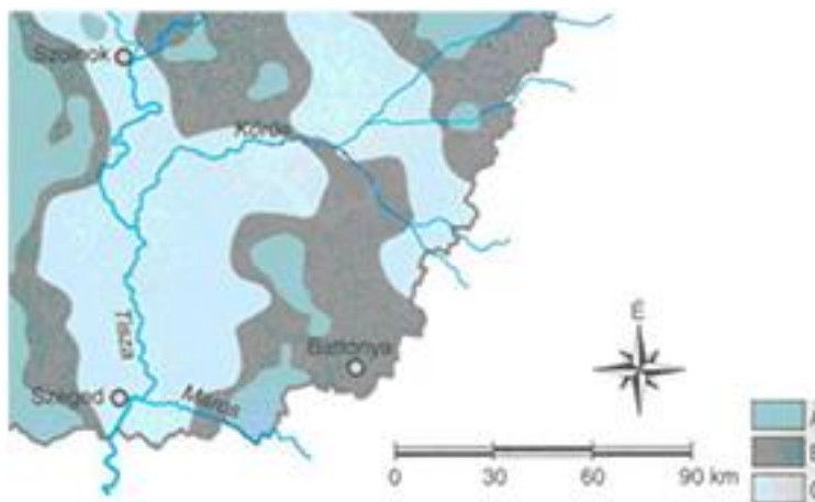
Felszín alatti vízár-rendszerek az Alföldön
