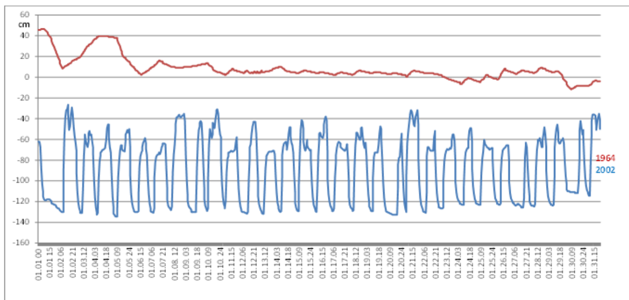
10. ábra: Vízjáték a Dráván januári hónapokban vízerőmű építés előtti és utáni időszakban
