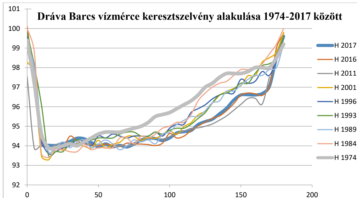
9. ábra: A Dráva keresztshelvényének változása a barcsi szelvényben
